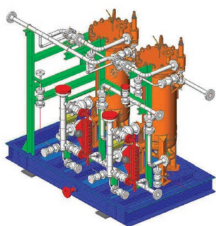
2019 SKID/VESSEL PER INSTALLAZIONE OFFSHORE RAVENNA
