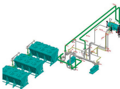
2019 MOSE BOCCA DI CHIOGGIA AVVIAMENTO MODALITÀ PROVVISORIA VENEZIA
